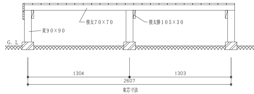
B 断面 図
