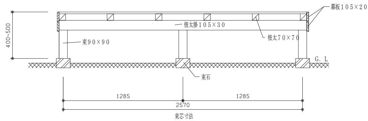
A 断面 図
